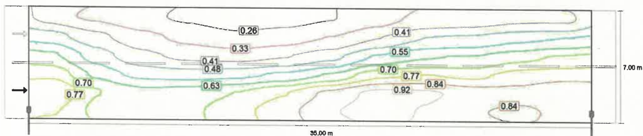
Observator 1: Densitatea luminii la instalația nouă [ \text{cd}/\text{m}^2 ] (Linii Isolux)
